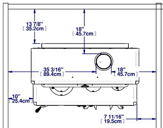
Distance au mur parois simple.
